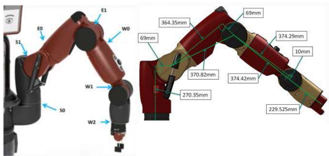
图附-1 机械臂关节分布示意
